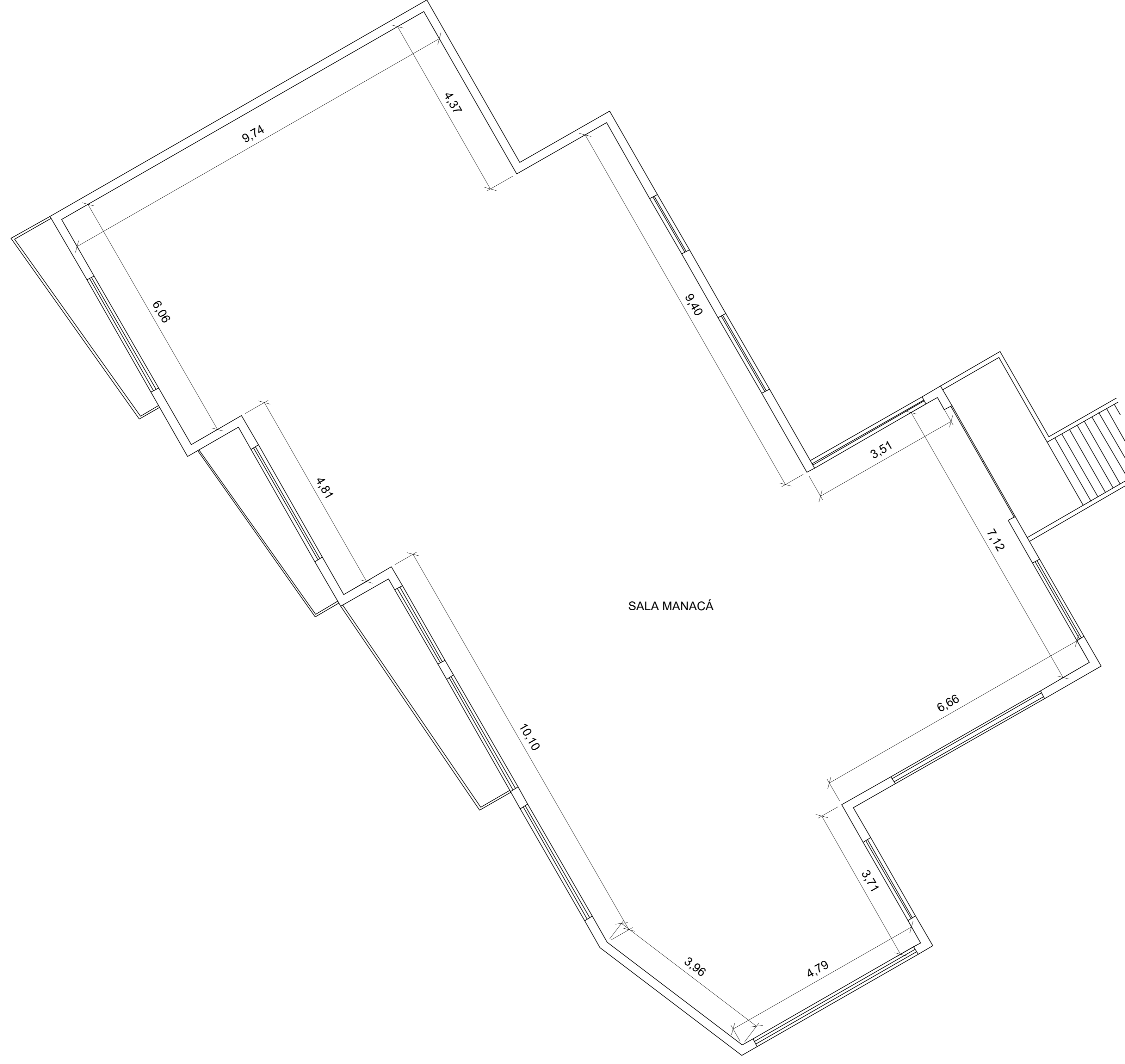
SALA MANACÁ - PISO BOI ESC. 1:100
